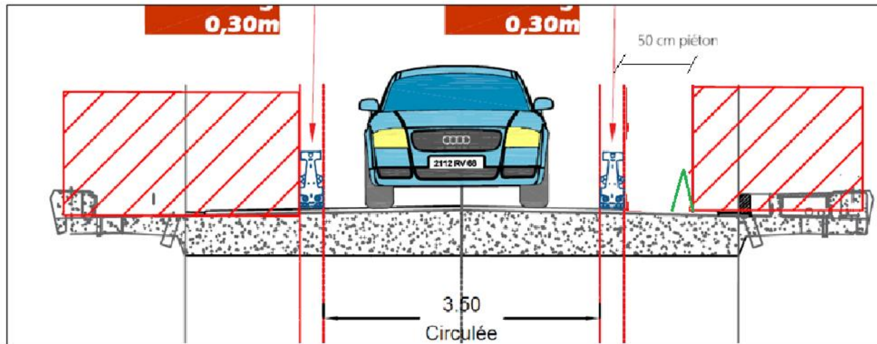
Figure 1 : Coupe du balisage. Cheminement piéton derrière cônes de chantier
